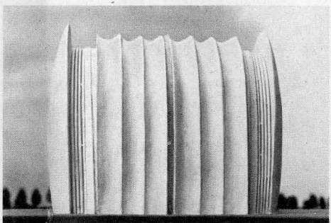
Projekt einer evangelischen Kirche aus vorgefertigten Stahlbetonschalen (Seite 629)
